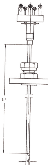
固定卡套法兰、可动卡套法兰 Fixed ferrule flange, Movable ferrule flange
