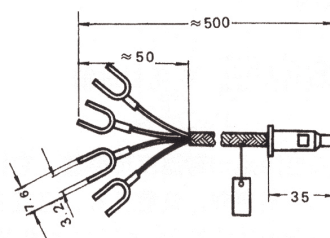
安装固定形式 Fixed installation
