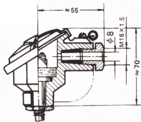
防溅式 接线盒 Splash proof junction box
