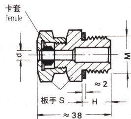
卡套螺栓式 Ferrule Bolt type
