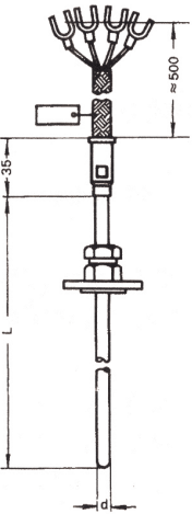
固定卡套法兰、可动卡套法兰 Fixed ferrule flange, movable ferrule flange
