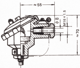
防水式 接线盒 water-proof junction box
